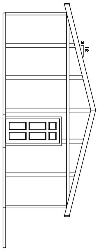
4 LEFT ELEVATION SCALE: 1/4" = 1'-0"
